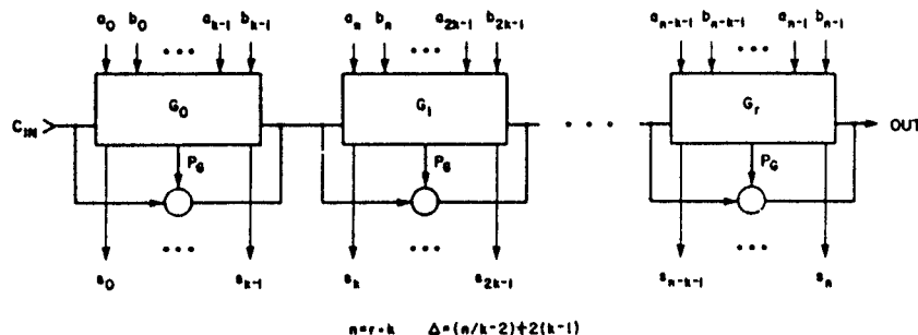
Fig.1. Carry-Skip Adder
